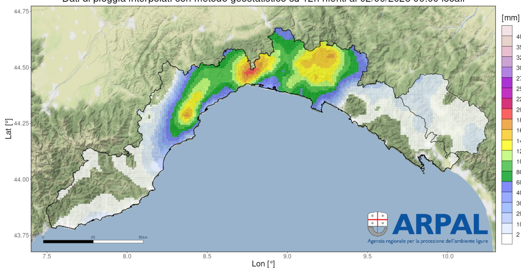
Dati di pioggia interpolati con metodo geostatistico su 12h riferiti al 02/09/2025 00:00 locali
